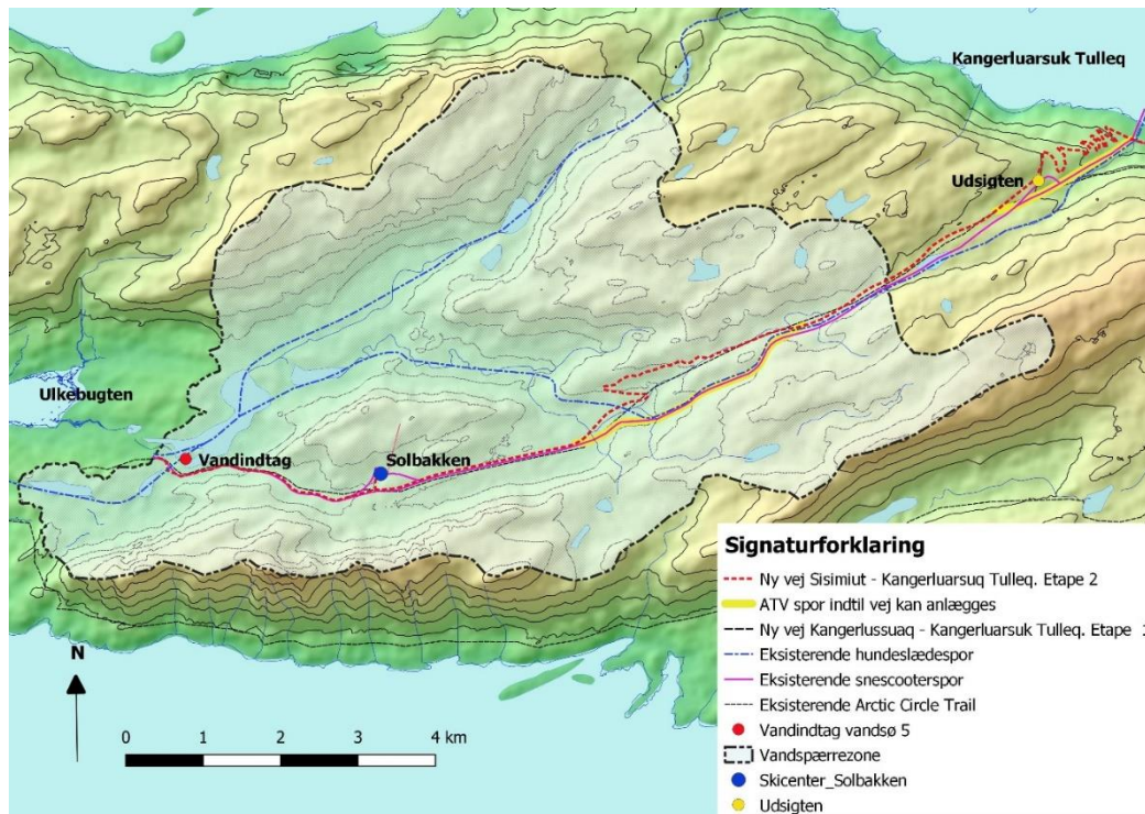
Ilusiliaq 1: Sisimiut aamma Kangerlussuaq akornanni aqutissatut pilersaarutigineqartoq. Ilusiliani takuneqarsinnaasutut, aqqusineq sumiiffimmi "Alannngorsuaq" aamma "Nasiffiup" akornanni sumiiffimmi ATV-t aqutissaannit allaanerussaaavoq.
