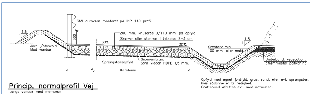
Ilusiliaq 2: Sanimut kipisaaq – taseq imeqarfik sinerlugu aqqusinniormissamut tunngaviusoq.
